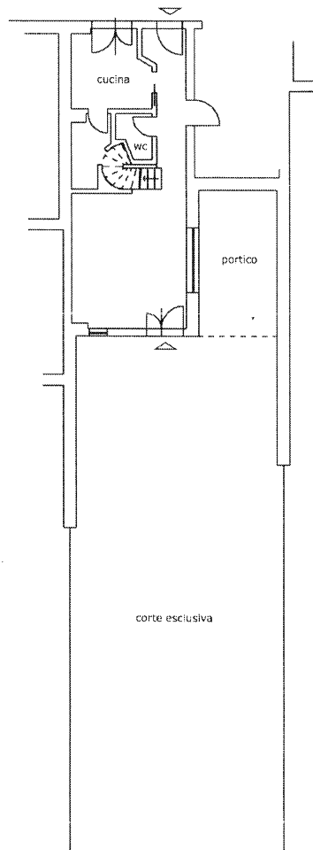
Pianta piano terra h= 2.70 m.
