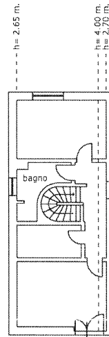
Pianta piano primo
